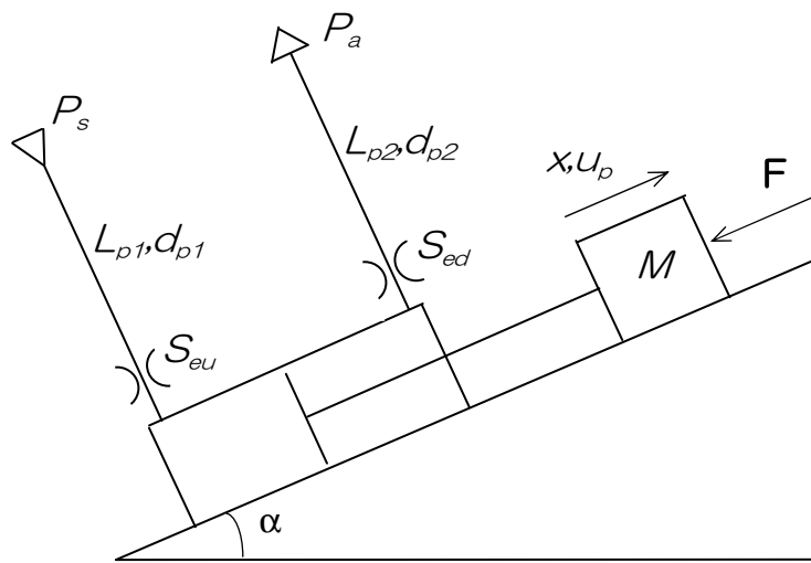
(a) システムモデル
