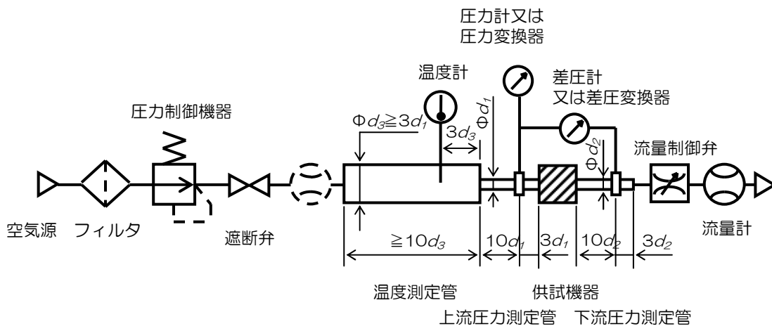
図2 ISO6358、JIS B 8390 の試験回路
