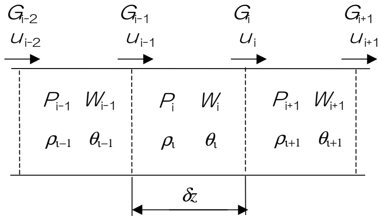
(b) 管路モデル
