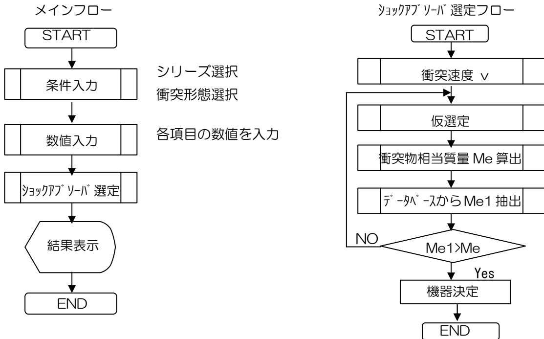
図 1 ショックアブソーバ選定プログラムの選定フロー
