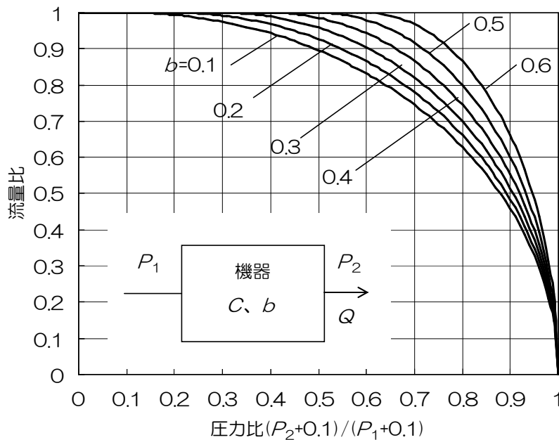
図 1 流量特性線図
