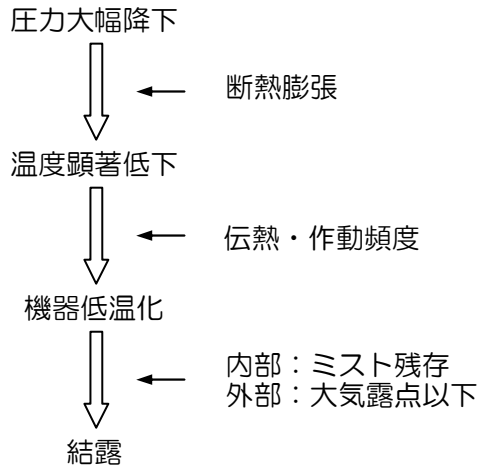
図2 機器表面の低温化による結露のメカニズム
