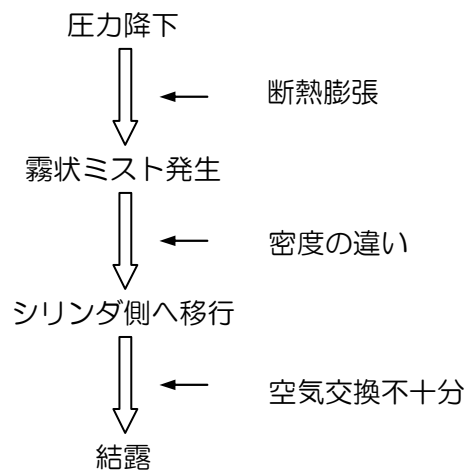
図1 空気交換不十分による結露のメカニズム
