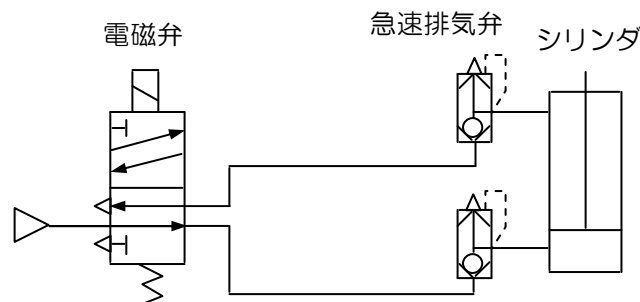
図3 急速排気弁による結露防止回路
