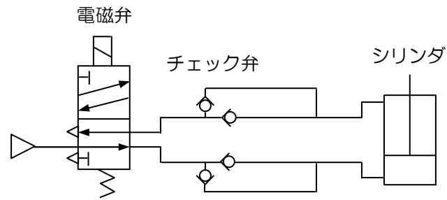
図4 バイパス管による結露防止回路
