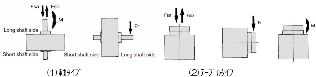
図 1 軸荷重
