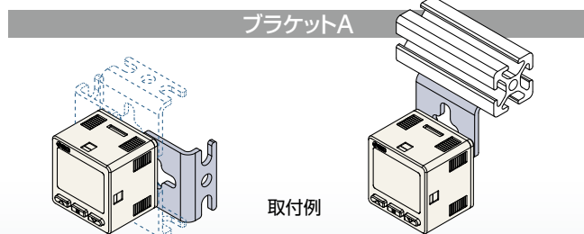
取付例
