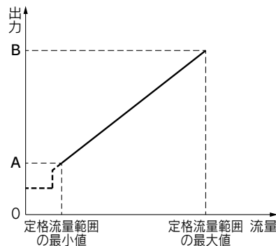
電圧出力 (1~5V) / 電流出力 (4~20mA)
