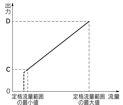
電圧出力 (0~10V)
