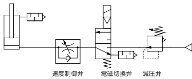
従来回路
