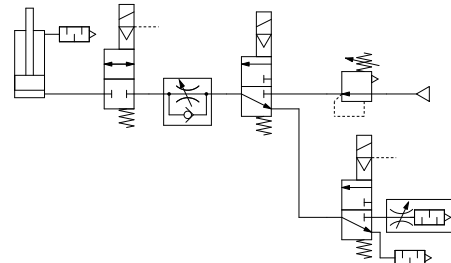
従来回路
