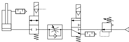
従来回路
