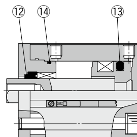
ø20, ø25
