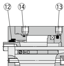
ø16
